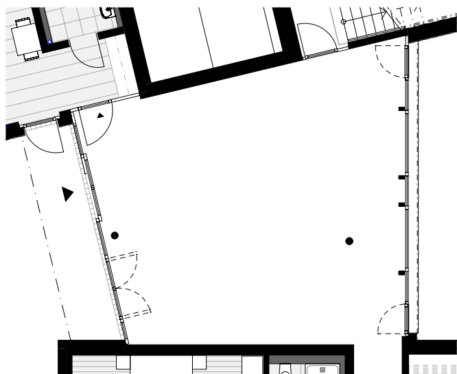
ERDGESCHOSS 1/150
