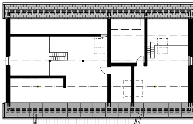
DACHGESCHOSS 1/150
