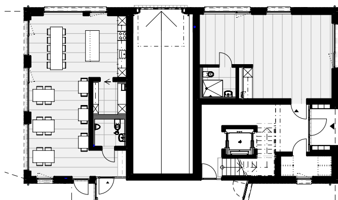
ERDGESCHOSS 1/150
