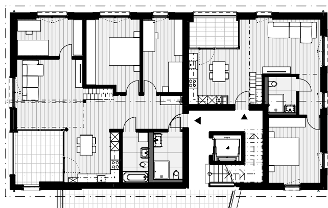
3. OBERGESCHOSS 1/150
