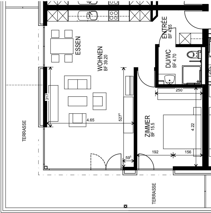
2 ½ ZIMMER - WOHNUNG MST. 1:100
