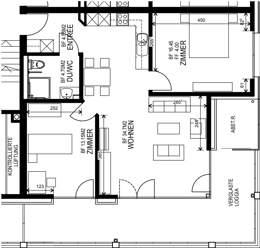
3 1/2 ZIMMER - WOHNUNG MST. 1:100
