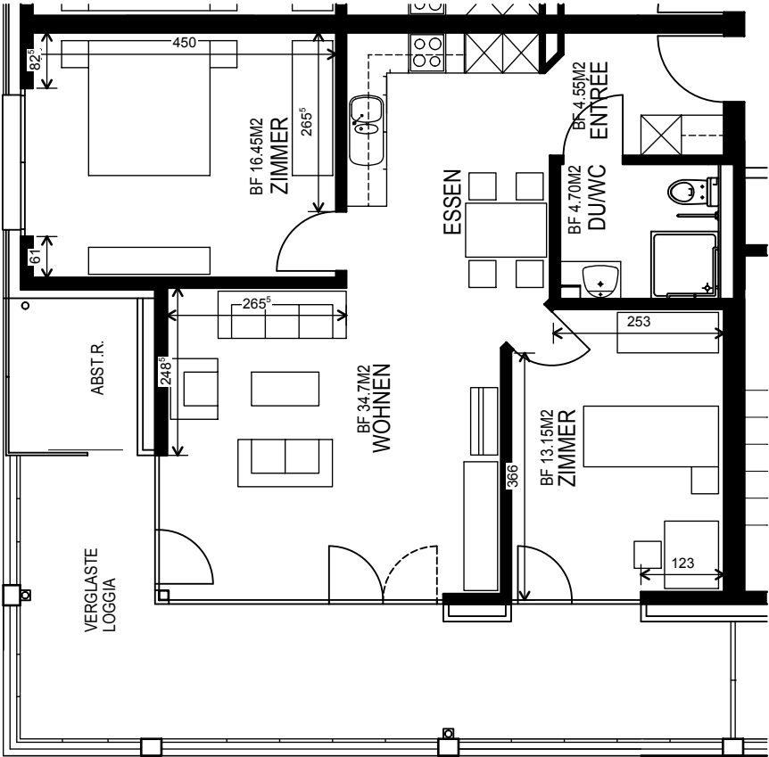
3 ½ ZIMMER - WOHNUNG MST. 1:100
